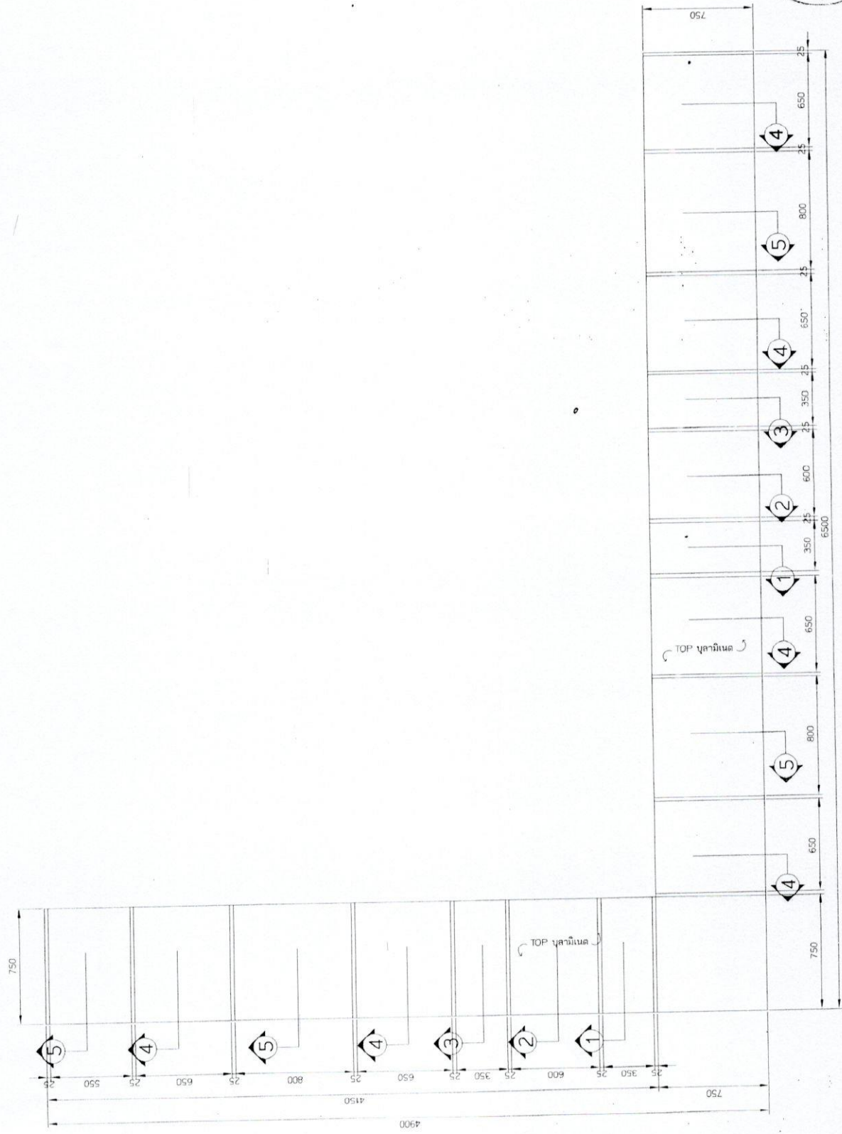
ขยายเคาน์เตอร์ พยาบาล SCALE 1:10
