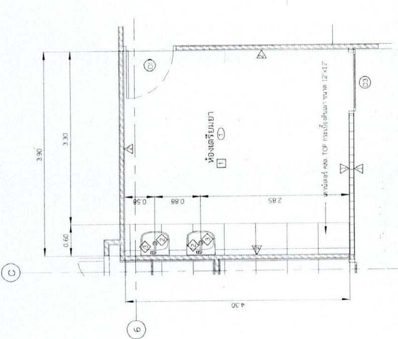
แผนพื้นที่ห้องเตรียมยา
